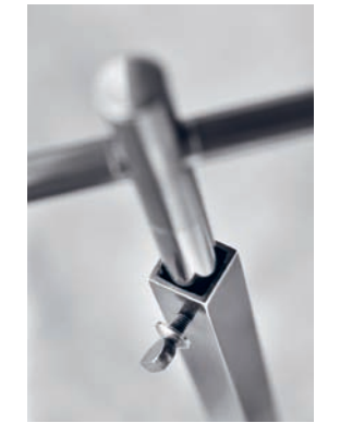
lampadaire télescopique avec réflecteur orientable en laiton patiné bronze | bronze patina moveable reflector and adjustable height
